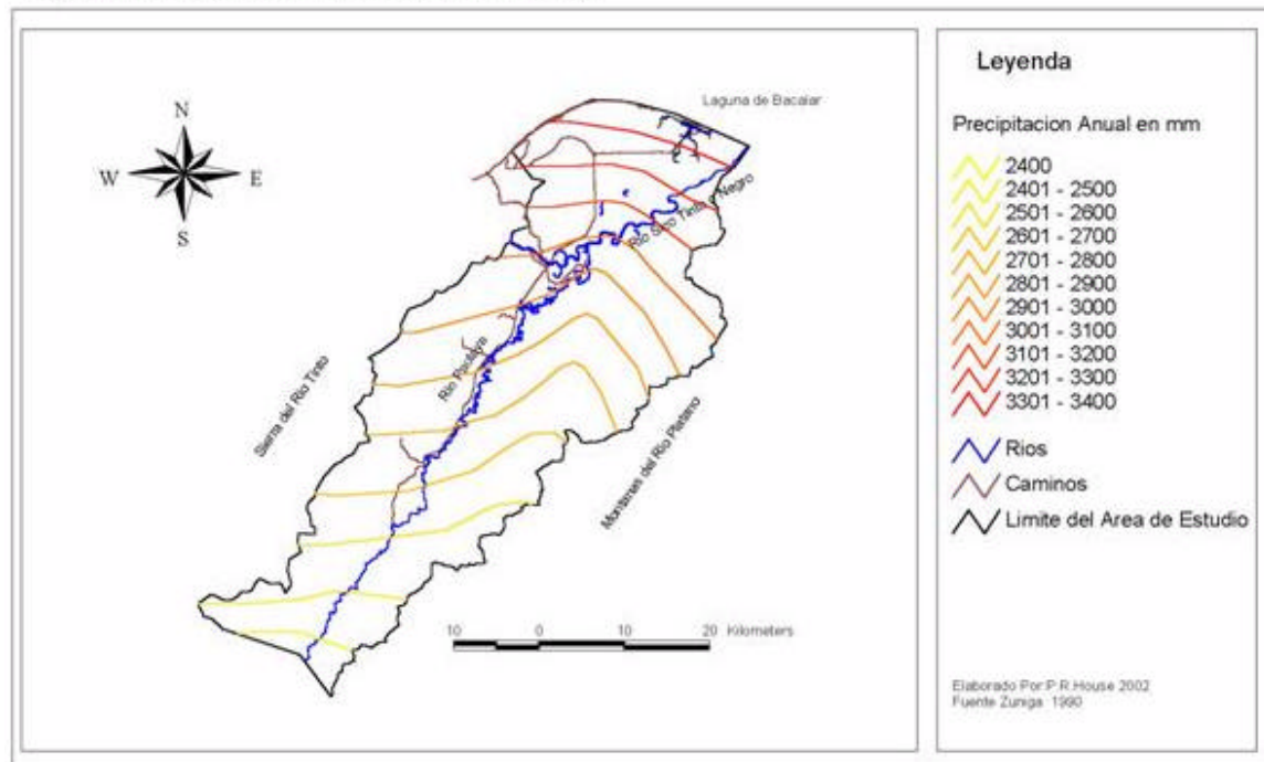
Mapa No. 6 Isohietas de Promedio de Lluvia Anual
