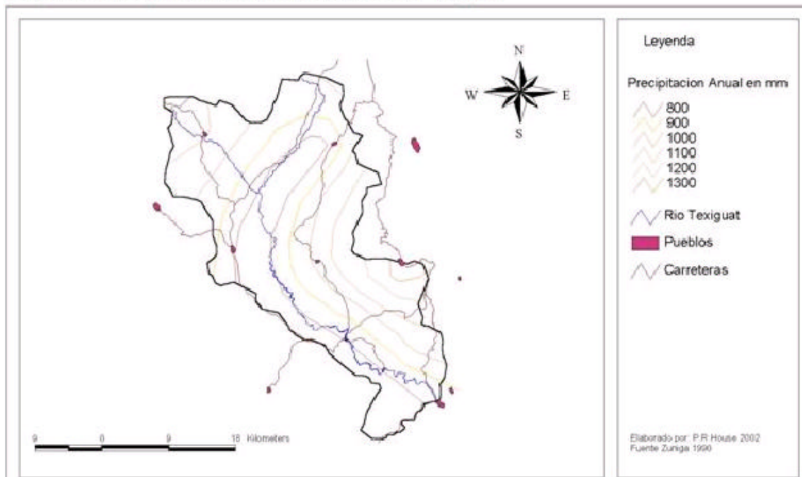
Mapa No. 6 Precipitación Anual en la Cuenca el Rio Texiguat
